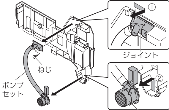
排水ポンプ
